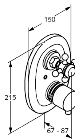
Размеры
